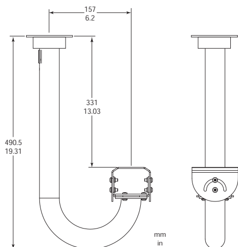
LTC 9219/01 J-vormige Montagebeugel voor Doorvoerbekabeling
