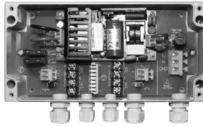
PSU-VAR-50W-2 (medium)
